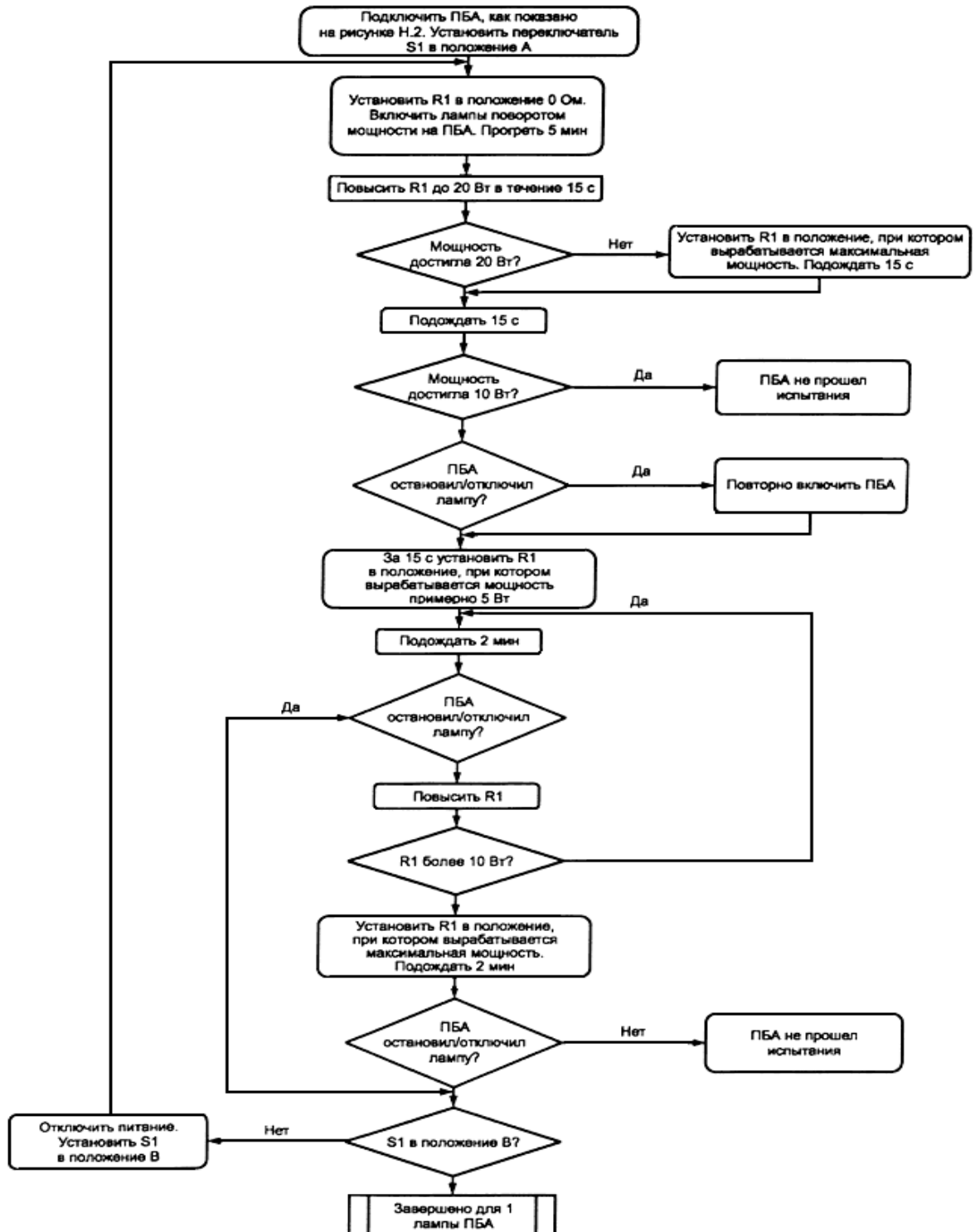
Рисунок Н.2 - Схема испытаний асимметричной мощностью
