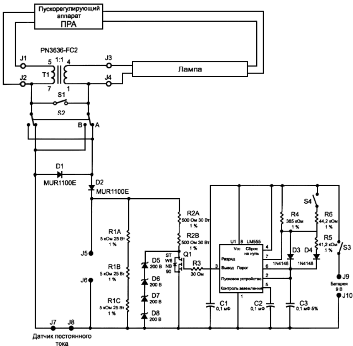
Рисунок Н.1 - Схема испытания асимметричным импульсом Пускорегулирующий аппарат должен быть присоединен к J2 и лампа к J4.
